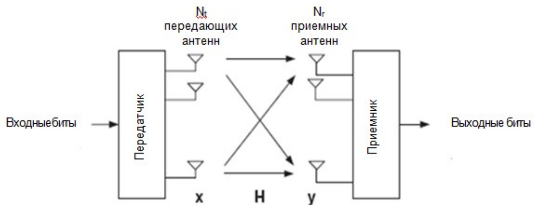
Рис.3.24. MIMO структура
