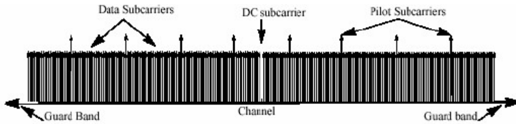
Рис. 3.18. Описание сигнала в частотной области
